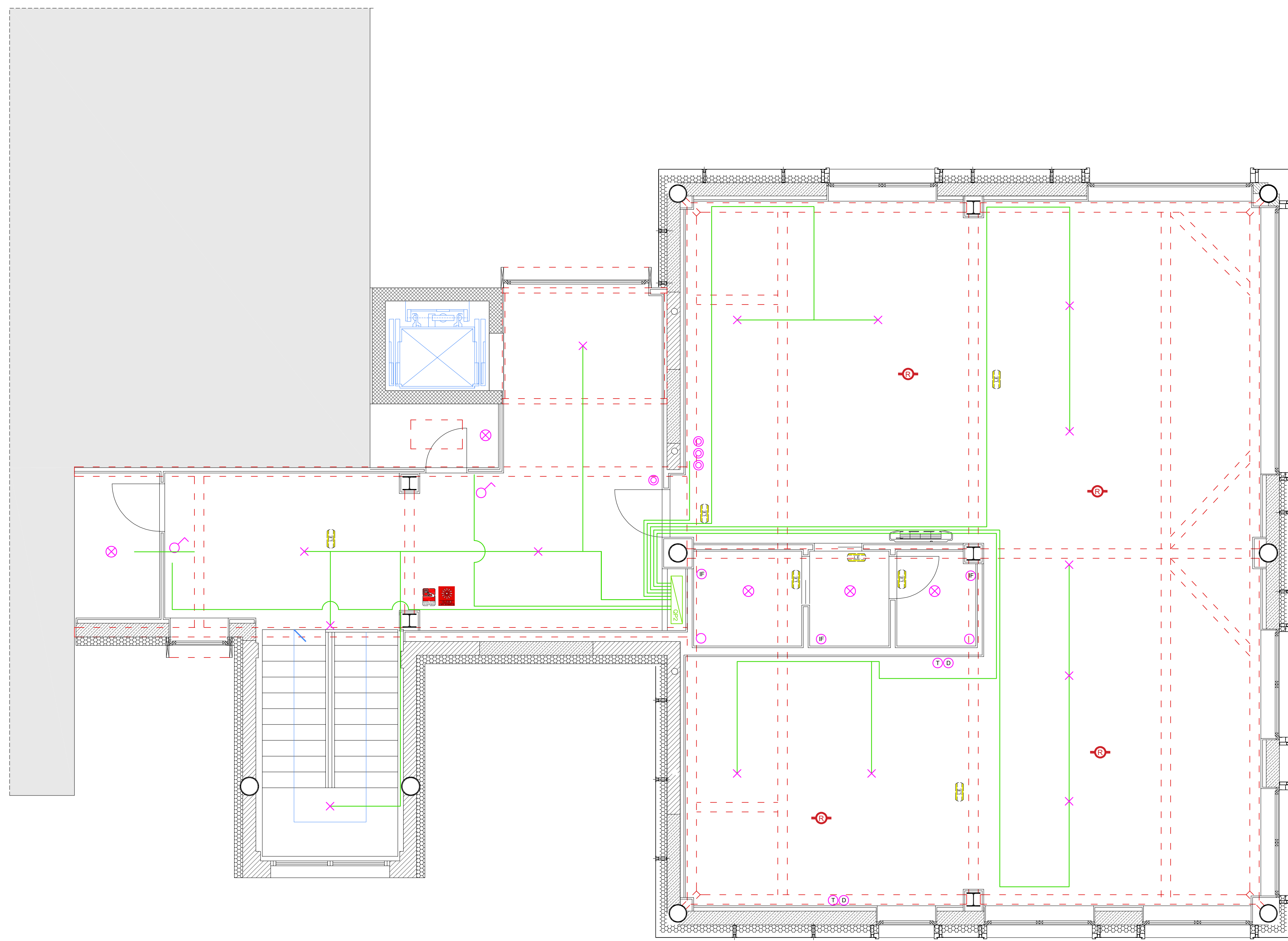
Stato di progetto - pianta piano secondo
