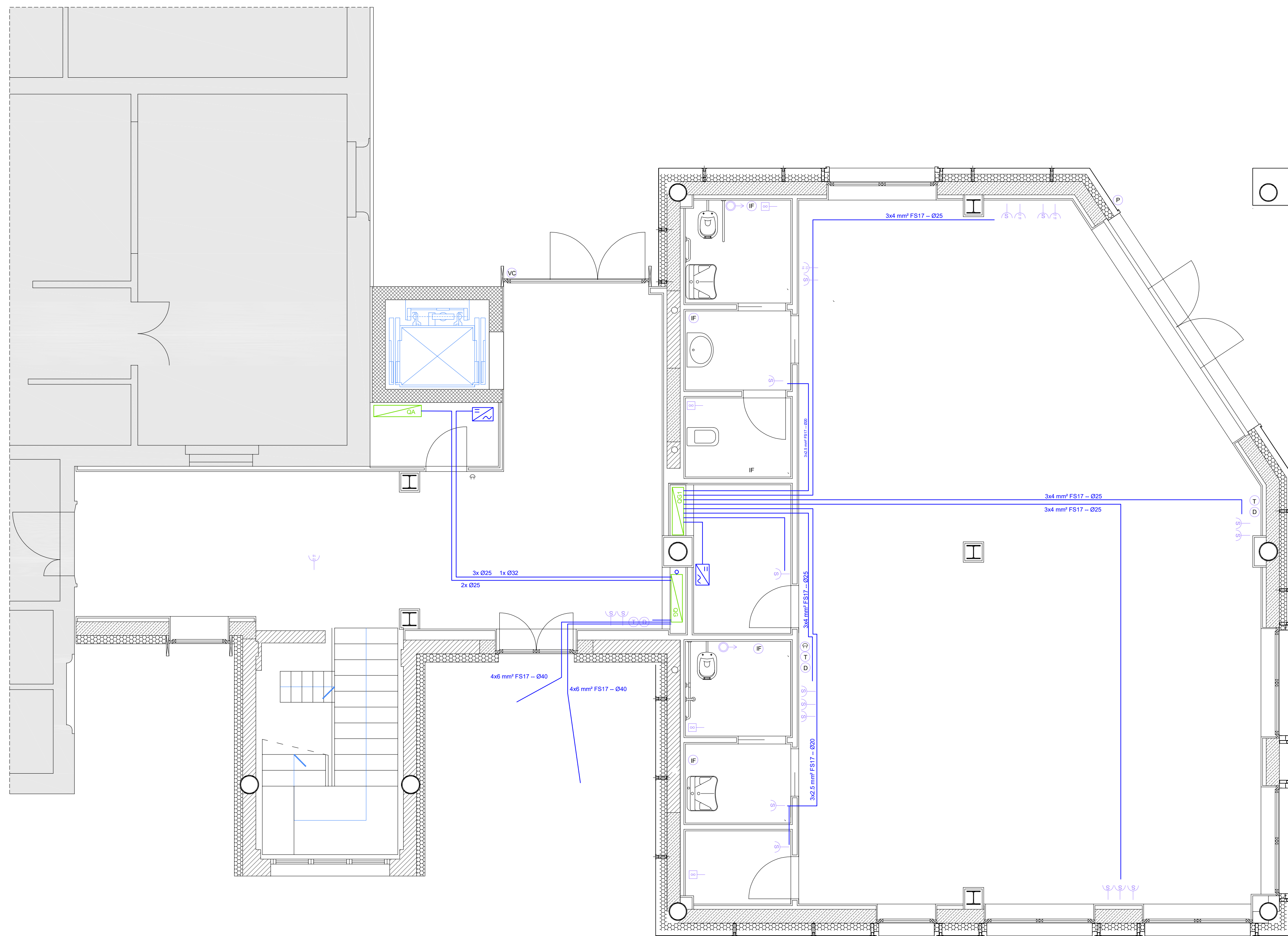
Stato di progetto - pianta piano terra
