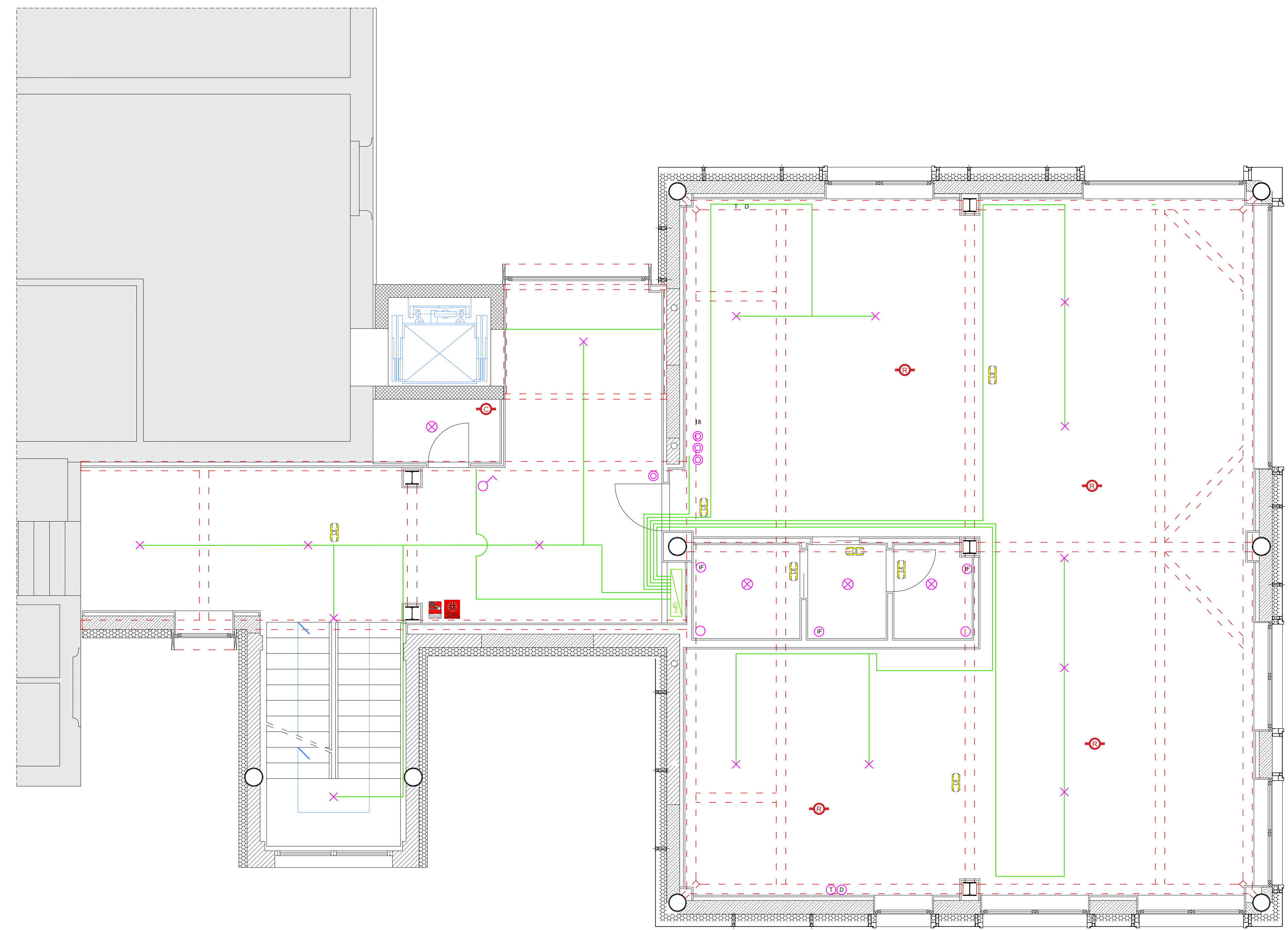
Stato di progetto - pianta piano primo
